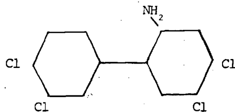
3',4,4',5-tetrachloro-2-biphenylamine
