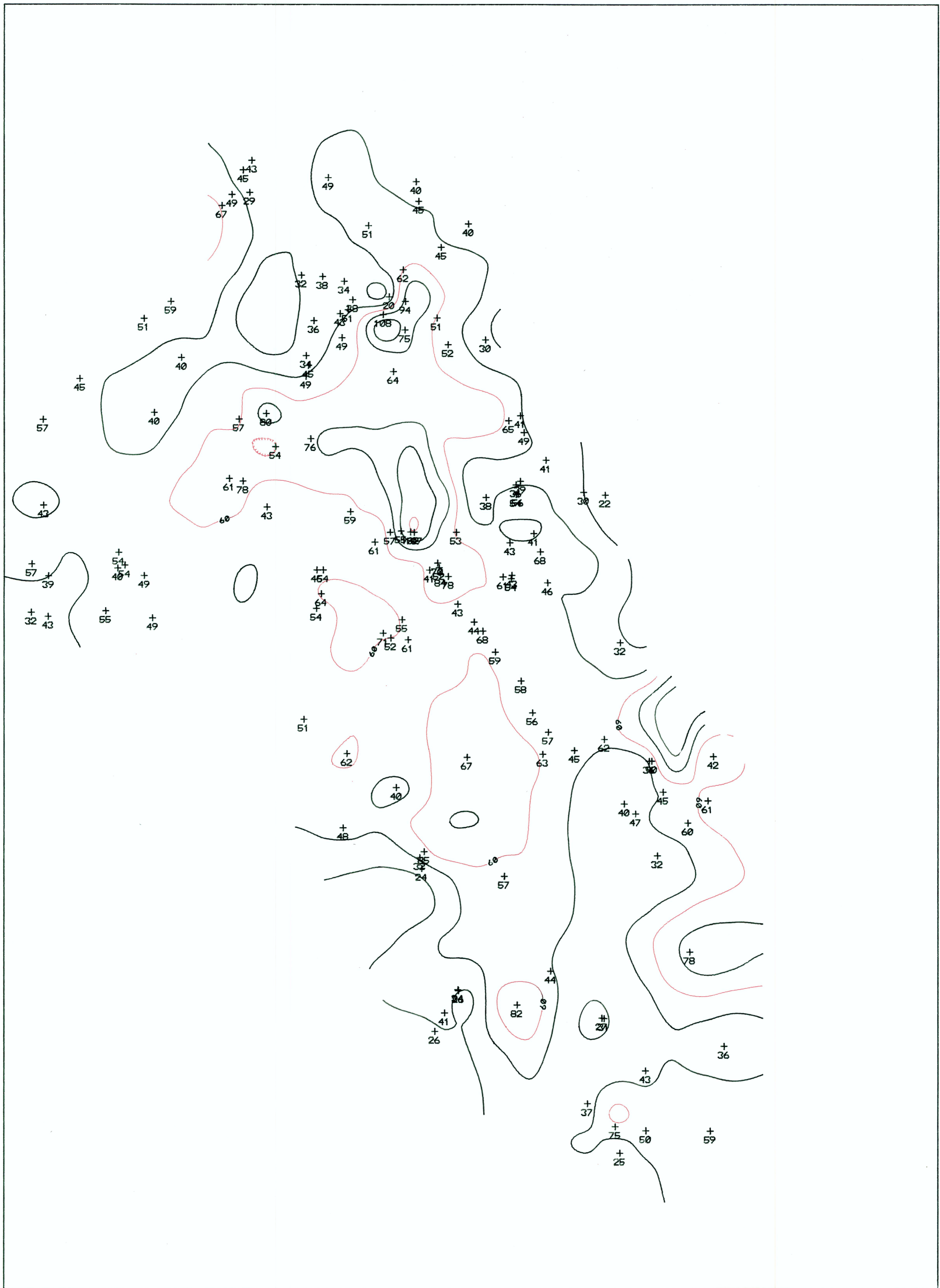
SILICA (SiO2)
