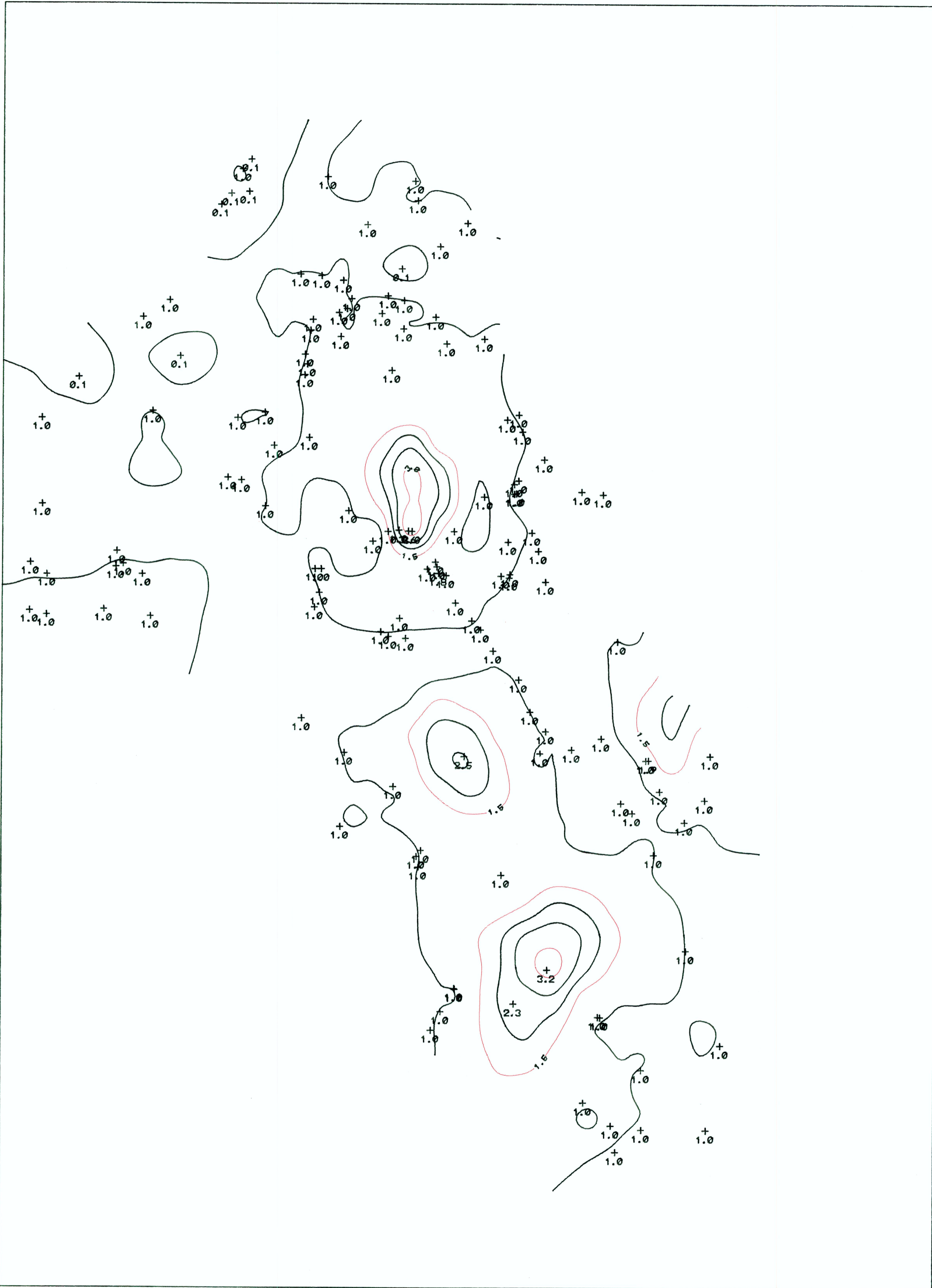
BORON ( B )
