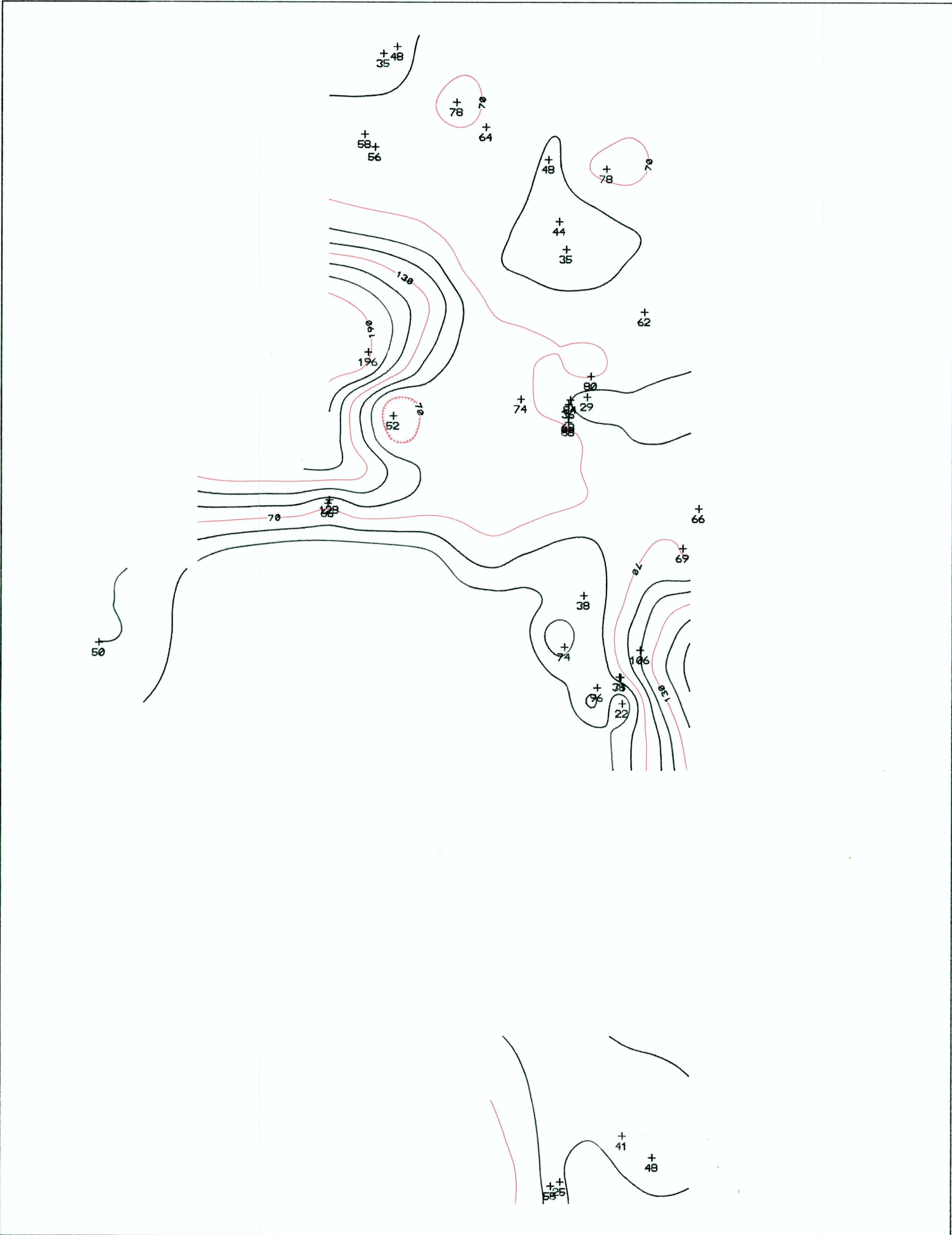
SILICA (SI02)
